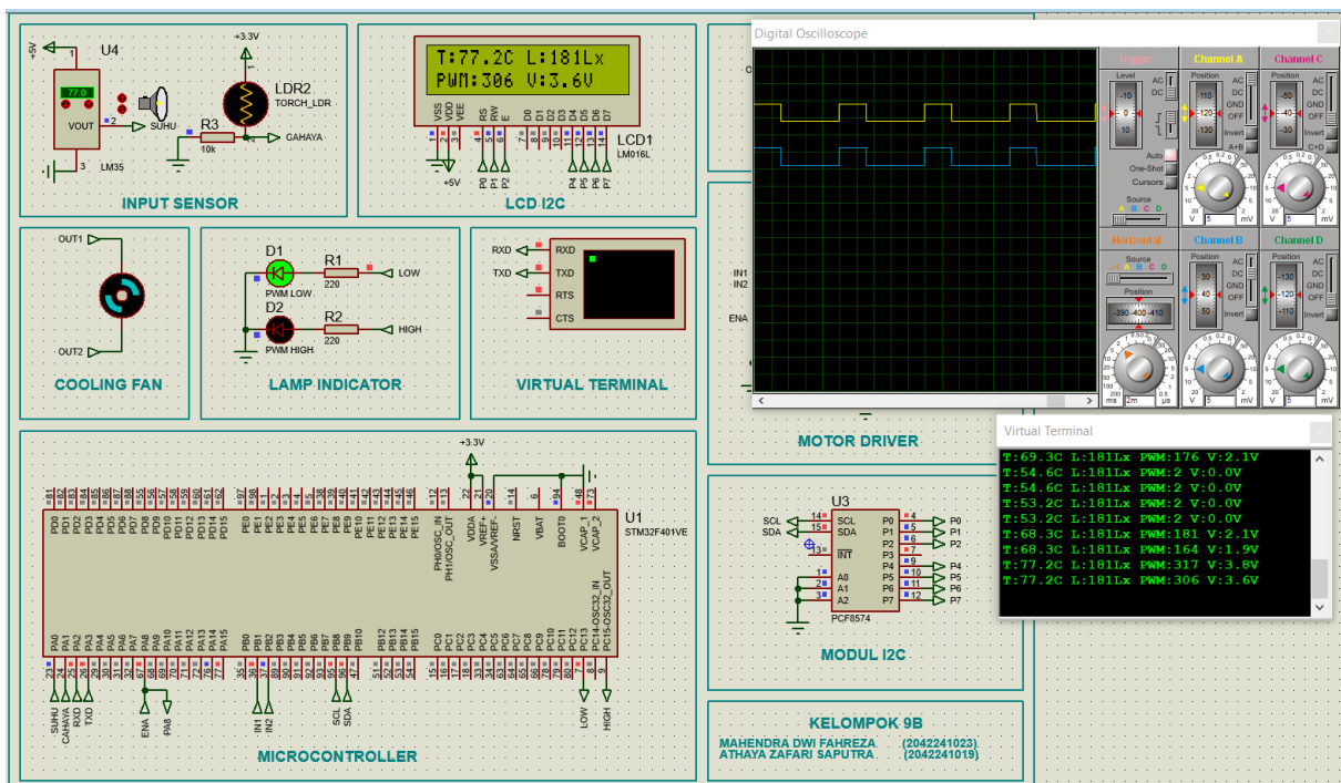
Figure 9: Tampilan keseluruhan simulasi pada kondisi operasi aman ( T = 77,2^{\circ}\text{C} ).
