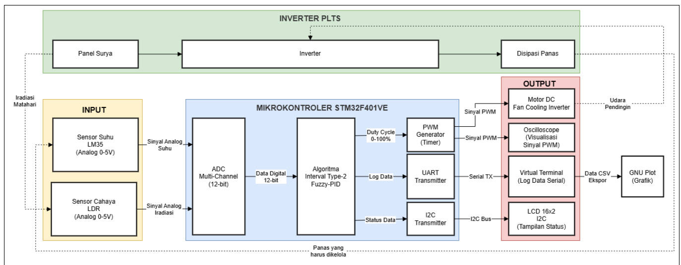
Figure 1: Diagram Blok Arsitektur Simulasi Software-in-the-Loop Sistem Manajemen Termal Interval Type-2 Fuzzy-PID pada Inverter PLTS Berbasis STM32F401VE.
