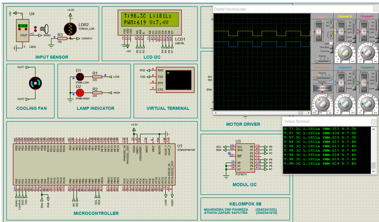
Figure 11: Tampilan keseluruhan simulasi pada kondisi suhu kritis ( T = 98,3^{\circ}\text{C} ).
