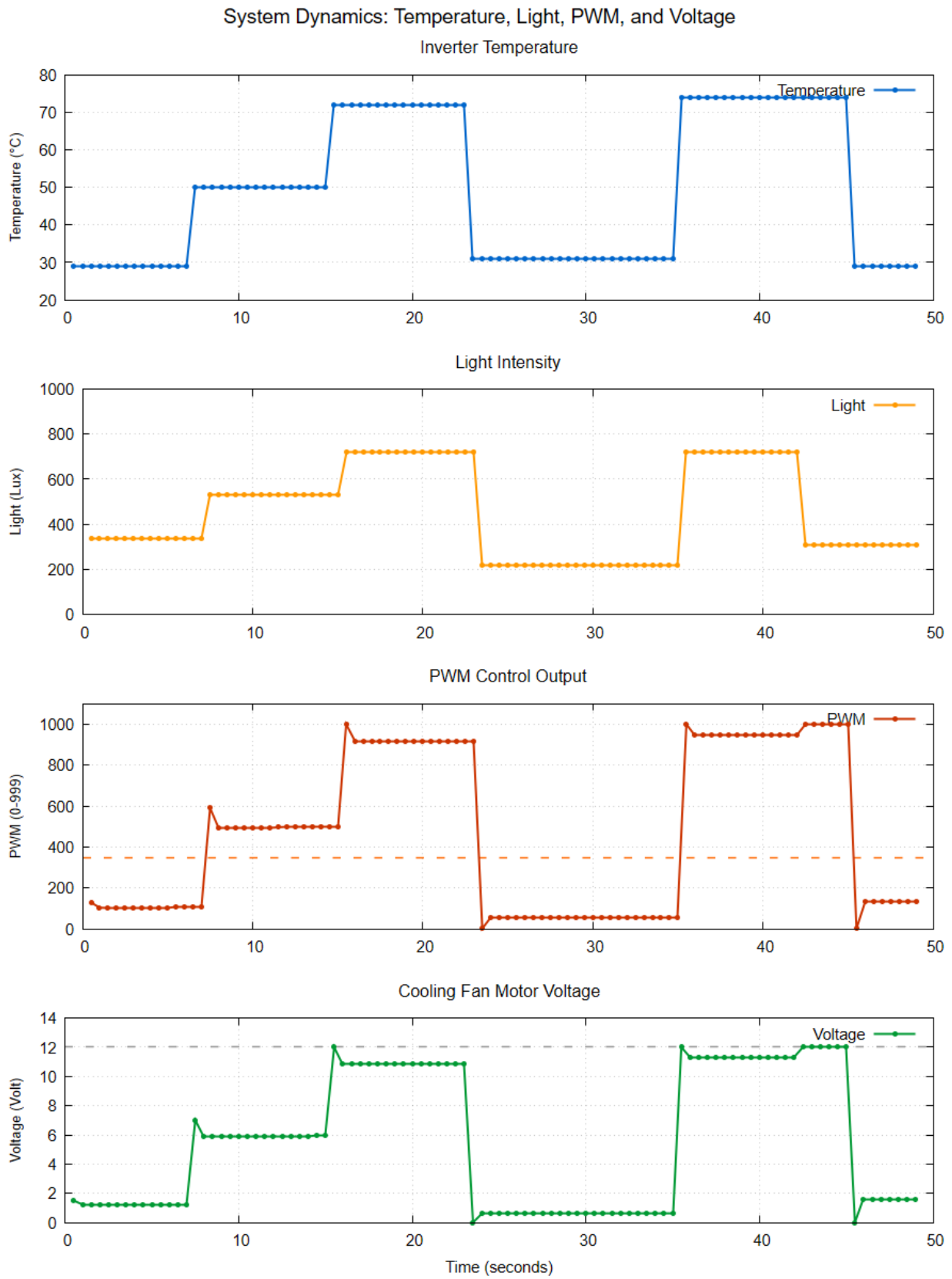
Figure 13: Multiplot dinamika waktu: Suhu aktual, Intensitas Cahaya, Respons PWM, dan Tegangan Motor.
