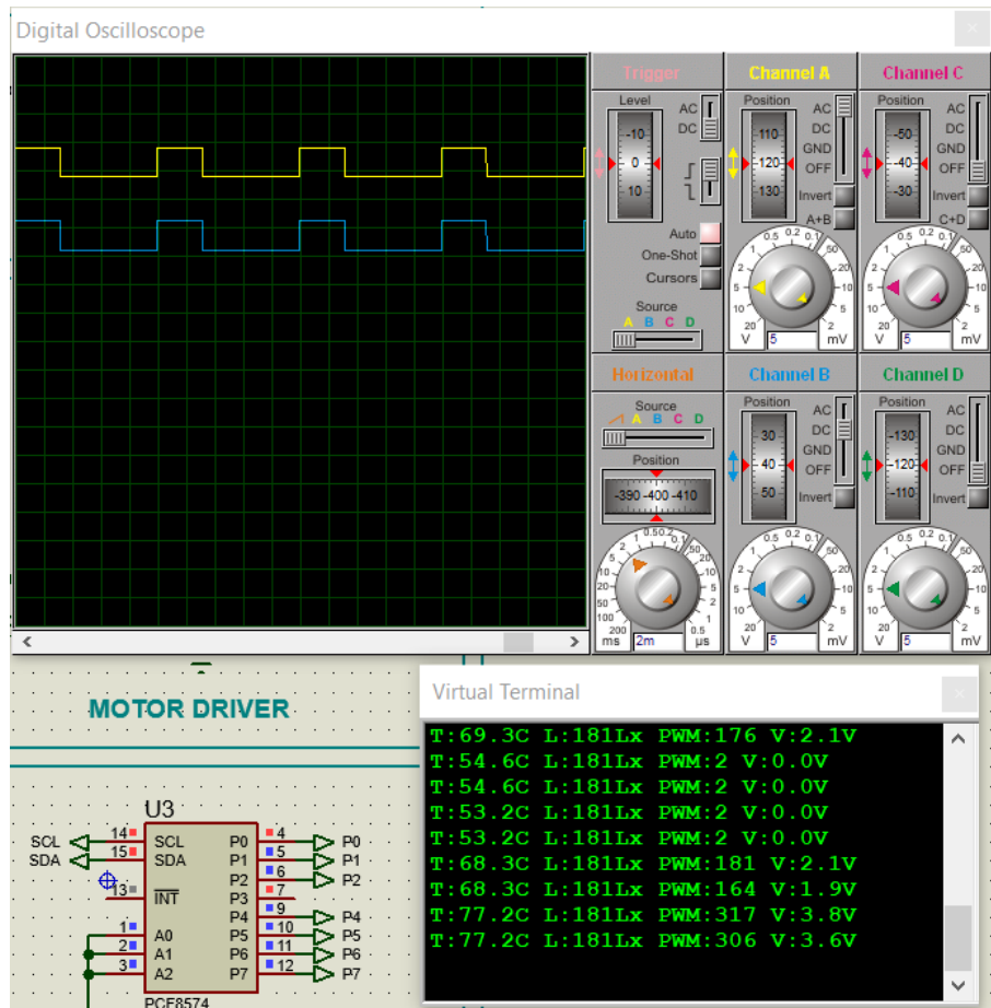
Figure 10: Virtual Terminal dan Oscilloscope pada kondisi operasi aman.
